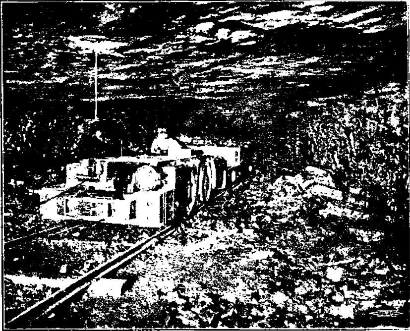
Kuuden tonnin sähköveturi tuo hiilijunaa kaivoksen etäisistä lokeroista.
