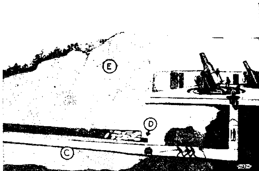
A. piirittäjien lähenevät juoksuhaudat; B, hyökkääjien tunneli; D, heldän asettamansa räjähdysaineet vallin alle; C, piiritettyjen puolustustunneli; E, kongreettinen puolustusvalli.
